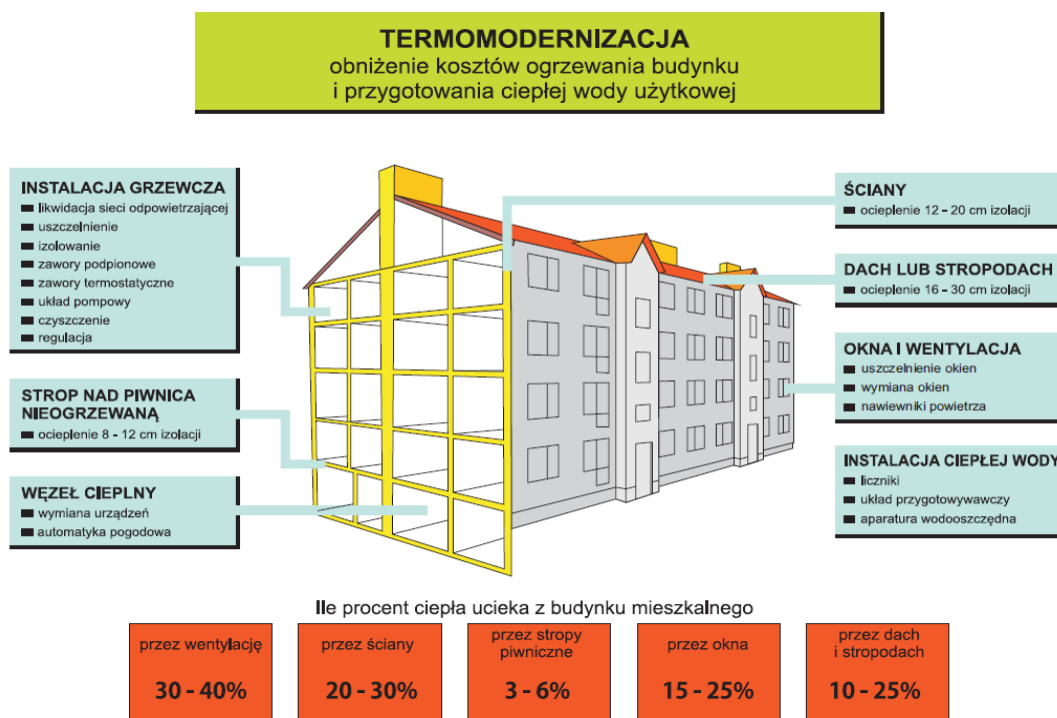
Ryc. 9. Termomodernizacja budynku
